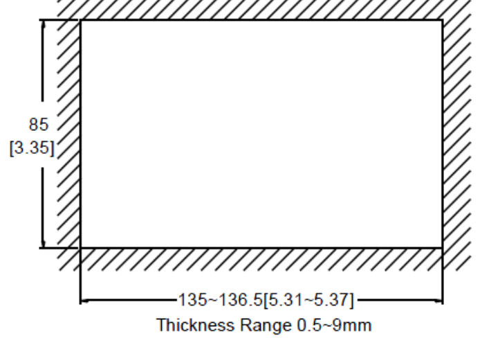
Montaj boyutları (birim: mm [inch])
